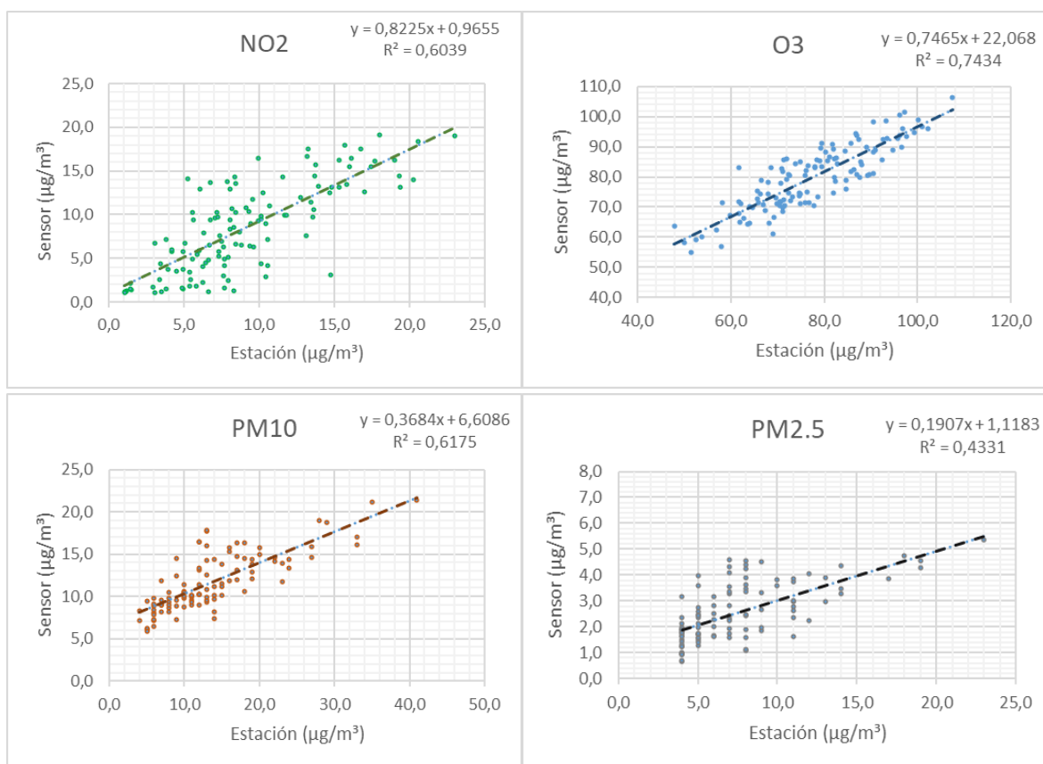
Ilustración 18. Correlación entre las mediciones del sensor y la estación homologada del Gobierno de Aragón, ubicados en el IES Sierra de Guara de Huesca. Fuente: Elaboración propia.
