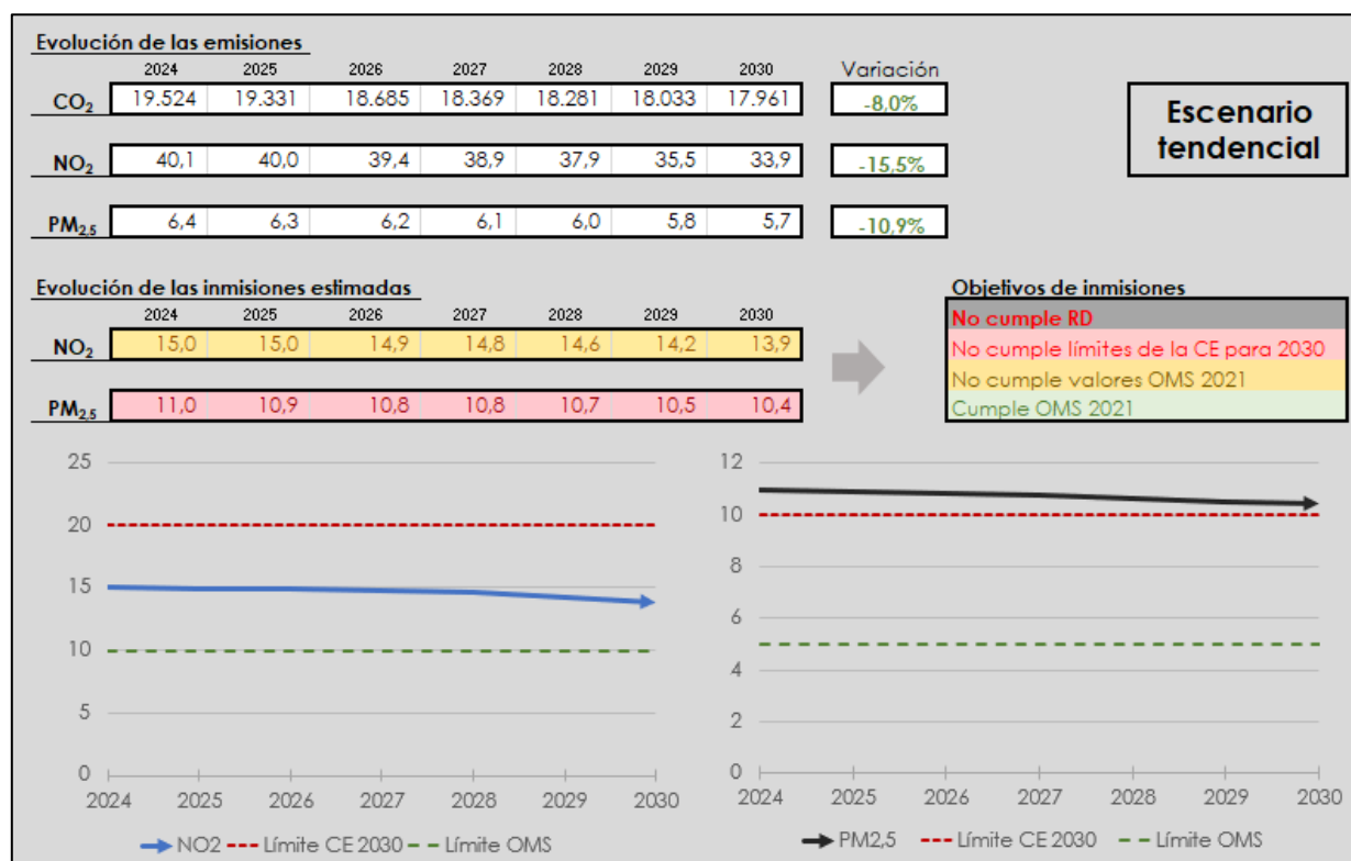
Ilustración 55. Estimación de la evolución de las emisiones de tráfico en Huesca (en toneladas), así como su afección en las inmisiones ( \mu\text{g}/\text{m}^3 ), según el escenario tendencial. Fuente: Elaboración propia.
