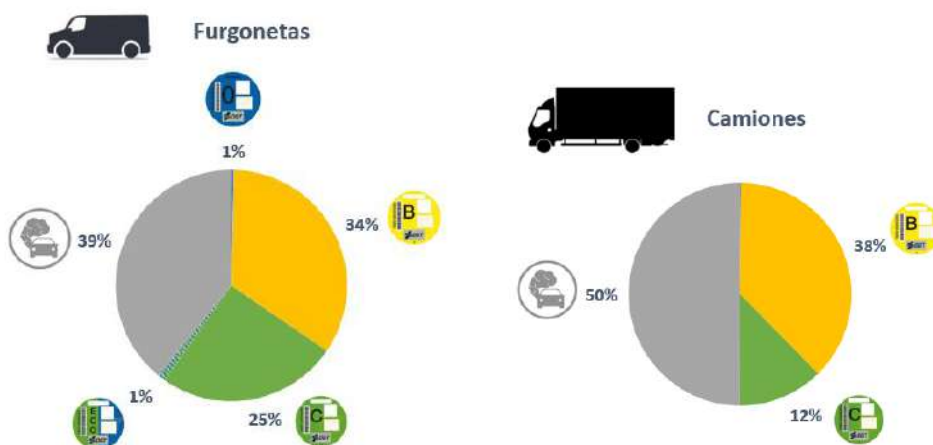
Ilustración 32. Composición del parque censado de vehículos comerciales (furgonetas y camiones) en Huesca en 2022. Fuente: DGT.
