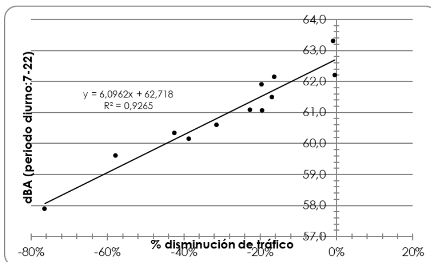
Ilustración 53. Relación entre nivel sonoro y tráfico en la ciudad de Madrid (2020). Fuente: Informe Estado de la Movilidad 2020 del Ayuntamiento de Madrid.
