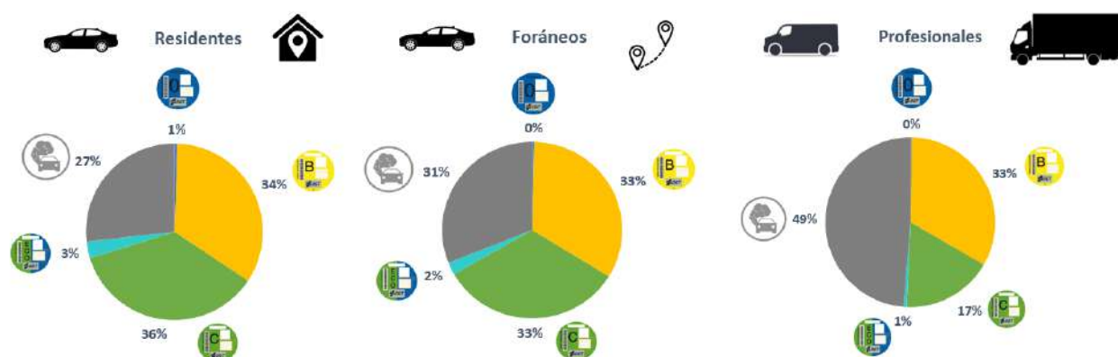
Ilustración 34. Distribución por distintivos ambientales de los vehículos del parque circulante de Huesca en 2022. Fuente: Elaboración propia a partir de datos de la DGT.
