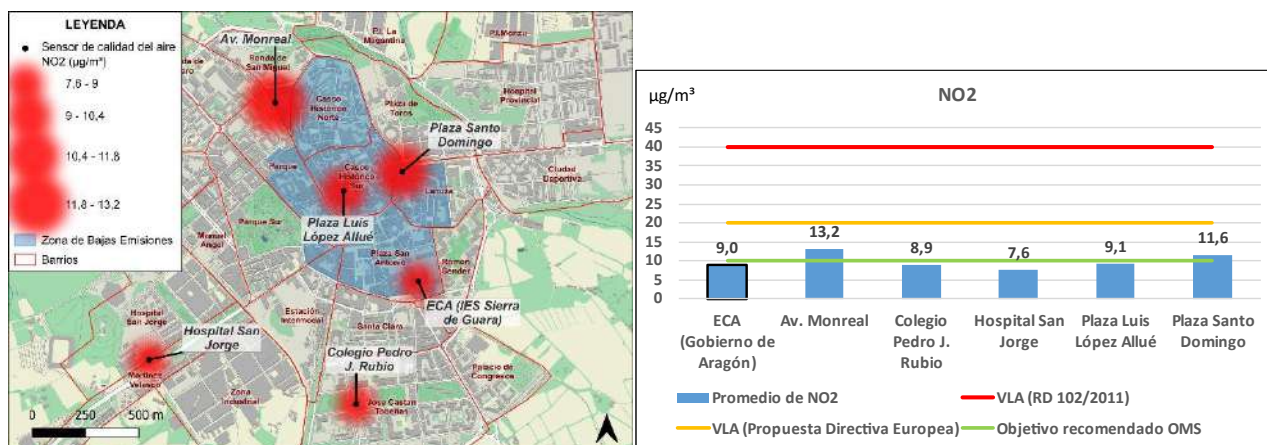
Ilustración 19. Promedio de dióxido de nitrógeno (µg/m 3 ) registrado por la Estación de Calidad del Aire (ECA) del Gobierno de Aragón y los sensores de calidad del aire entre abril y agosto de 2024. Fuente: Elaboración propia.
