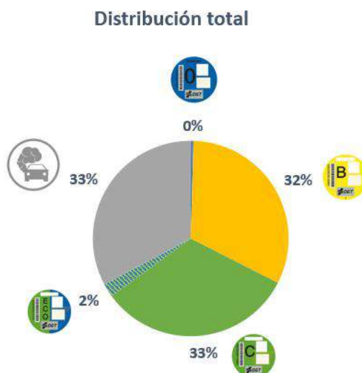
Ilustración 30. Composición del parque censado según distintivo ambiental en Huesca en 2022. Fuente: DGT.
