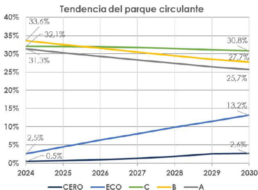
Ilustración 54. Tendencia esperada en la transformación del parque circulante en Huesca. Fuente: Elaboración propia.
