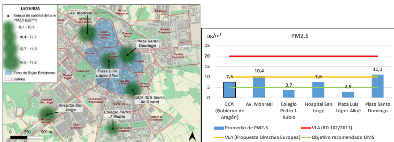
Ilustración 22. Promedio de partículas PM_{2,5} ( \mu g/m^3 ) registrado por la Estación de Calidad del Aire (ECA) del Gobierno de Aragón y los sensores de calidad del aire entre abril y agosto de 2024. Fuente: Elaboración propia.
