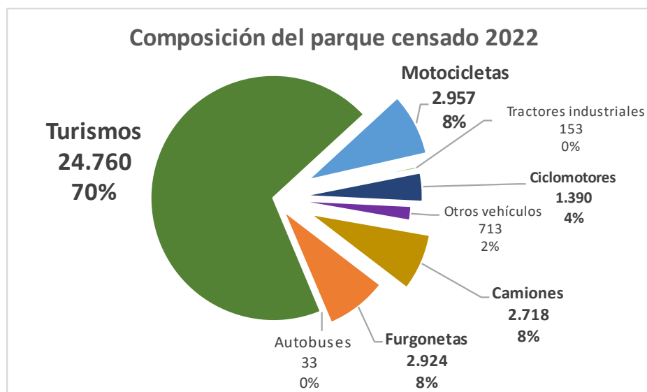
Ilustración 29. Composición del parque de vehículos censado según la tipología (2022). Fuente: DGT.
