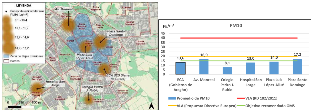
Ilustración 21. Promedio de partículas PM_{10} ( \mu g/m^3 ) registrado por la Estación de Calidad del Aire (ECA) del Gobierno de Aragón y los sensores de calidad del aire entre abril y agosto de 2024. Fuente: Elaboración propia.
