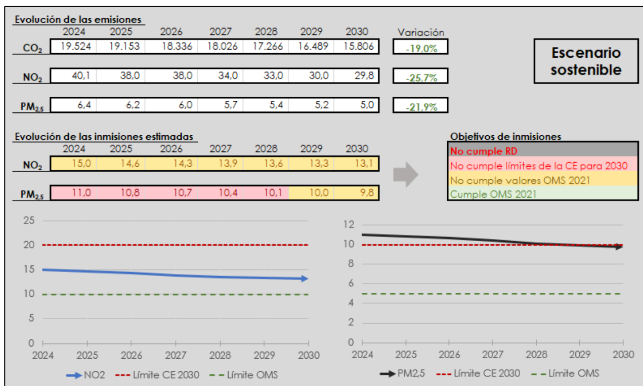
Ilustración 56. Estimación de la evolución de las emisiones de tráfico en Huesca (en toneladas), así como su afección en las inmisiones ( \mu\text{g}/\text{m}^3 ), según el escenario sostenible. Fuente: Elaboración propia.
