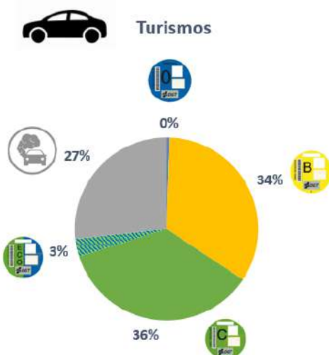
Ilustración 31. Composición del parque censado de turismos según distintivo ambiental en Huesca en 2022. Fuente: DGT.
