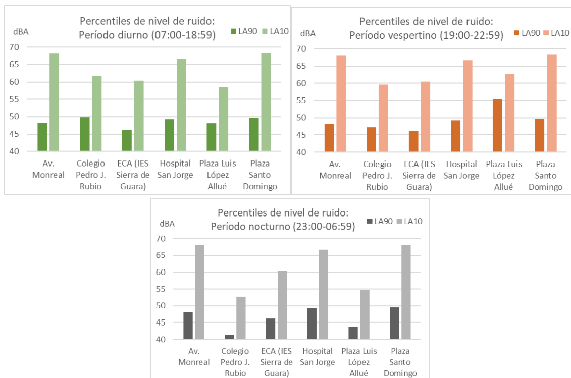
Ilustración 27. Percentiles de nivel de ruido ponderado A: percentil 90 (LA90) representando el ruido ambiente de fondo y percentil 10 (LA10) representando los eventos de mayor ruido. Valores promedio de los registros entre abril y agosto de 2024 en Huesca.
