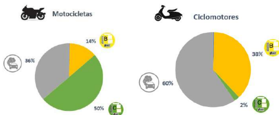
Ilustración 33. Composición del parque censado de vehículos de menor tamaño (motocicletas y ciclomotores) en Huesca en 2022. Fuente: DGT.
