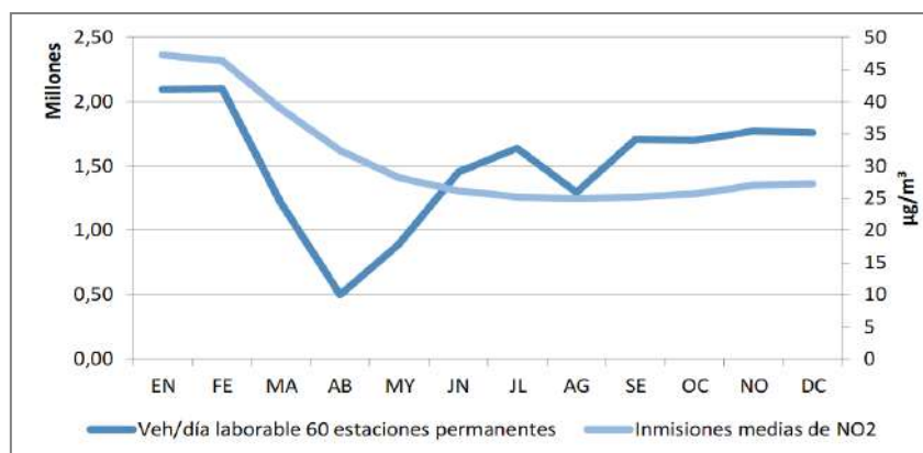
Ilustración 52. Relación de inmisiones de \text{NO}_2 y tráfico en la ciudad de Madrid (2020). Fuente: Informe Estado de la Movilidad 2020 del Ayuntamiento de Madrid.
